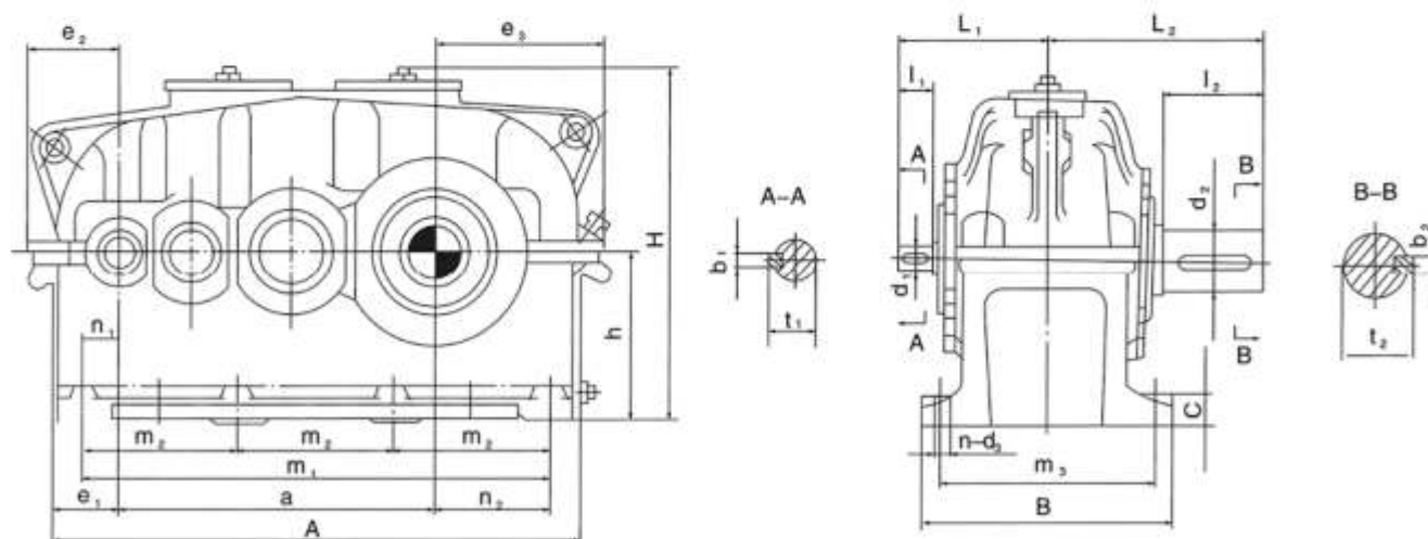
YFZSY、YFZSZ型装配型式
