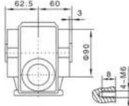
YFS..37R17
