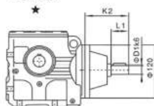
YFS..S37
