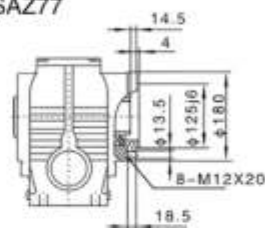
YFSAZ77
