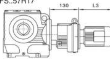
YFS..57R17
