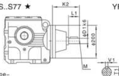
YFS..S77 ★
