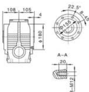
YFSAZ77
