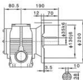
YFSF67
