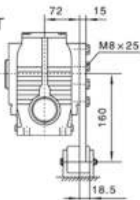
YFSA57/T
