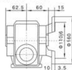
YFSAF37/Φ160
